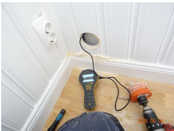
Bild 3: Fuktmätning av FK i vägg, Rum 1
