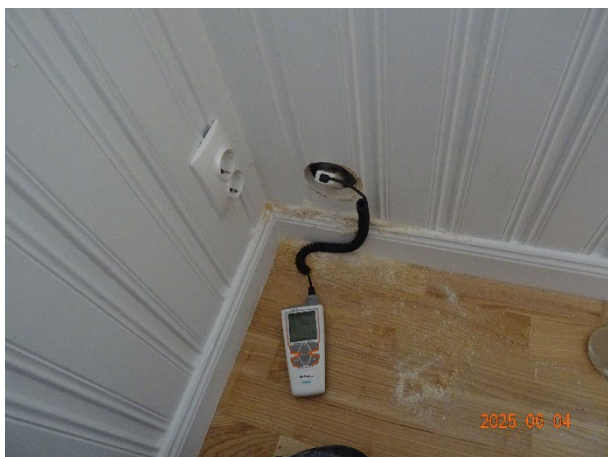
Bild 5: Fuktmätning av RF i golv, Rum 1
