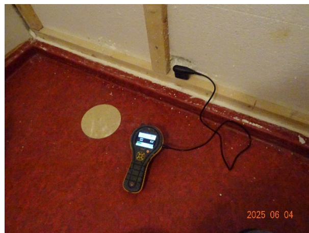
Bild 6: Fuktmätning av FK i vägg, förråd
